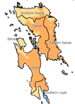
SPEI3 (Oct-Nov-Dec)
